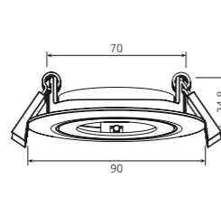
TILT TRIM Ø80
