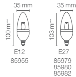
3W E12 Opalino 3W E27 Opalino 3W E27 Clear
