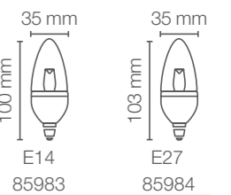
4W E14 4W E27
